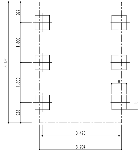
■ 基礎配置図
